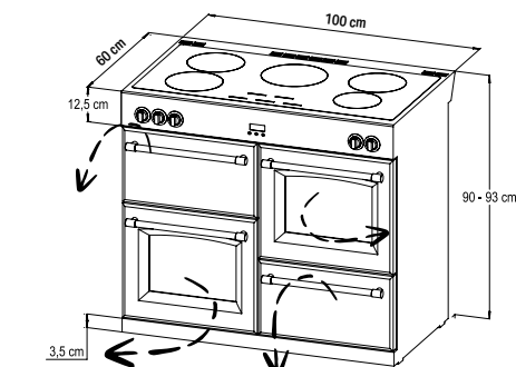
Richmond/Sterling S1000 Ei Richmond/Precision S1000 Ei
