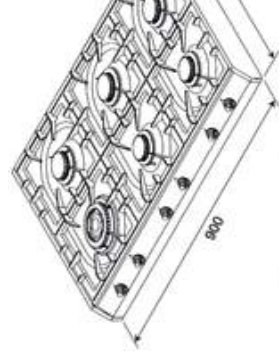
PGK 96 | GAS AANSluitING LINKS
