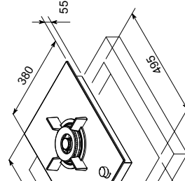
UITING RECHTS ACHTER
